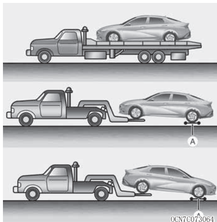
[A]: 移动台车
