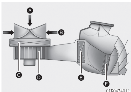
[A]: 空气外循环, [B]: 空气内循环 [C]: 空调滤清器, [D]: 鼓风机 [E]: 蒸发器芯, [F]: 加热器芯
